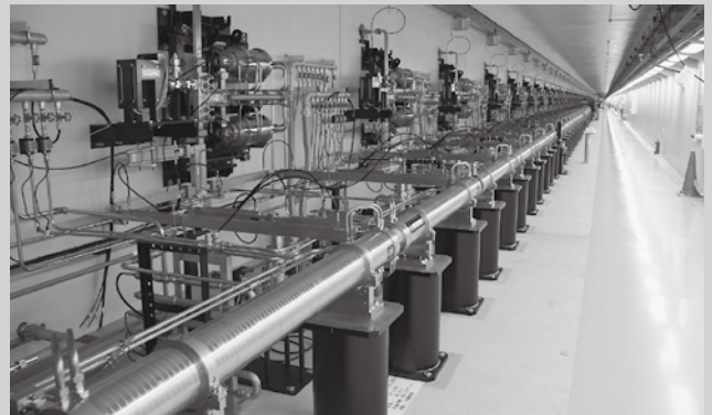
SACLAの加速器棟トンネル内に並ぶ128本のCバンド加速管
