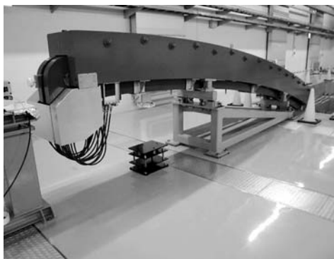
レーザー発振後、電子を取り除く 全長7 mのXFELダンプ電磁石
