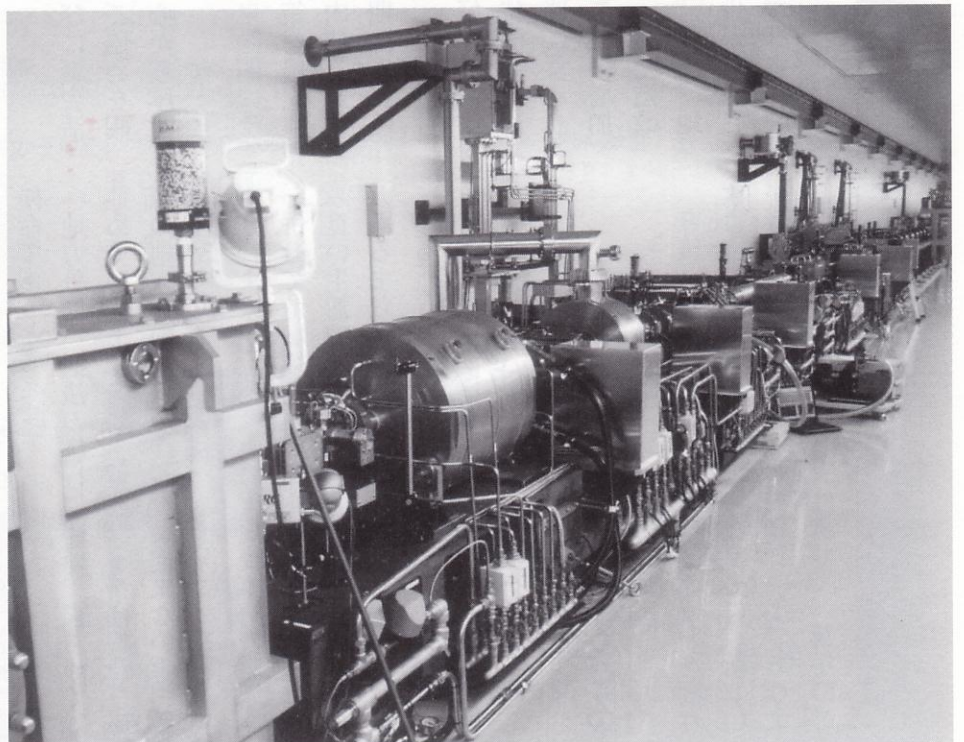
現在スプリング8サイト内にある延長約60mの試作機（プロトタイプ機）
