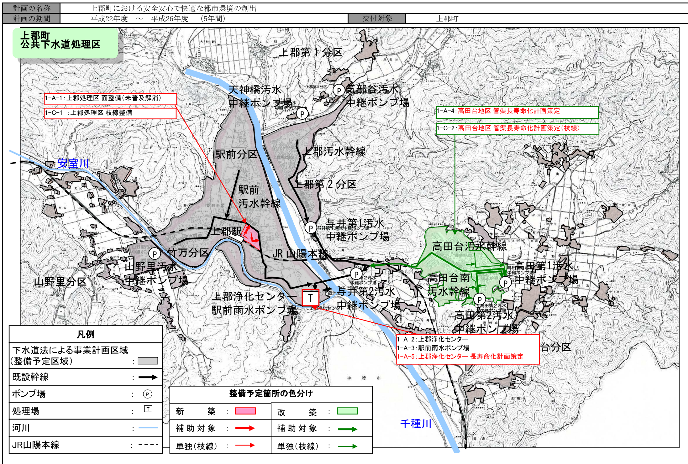
(図面) 水の安全・安心基盤整備
